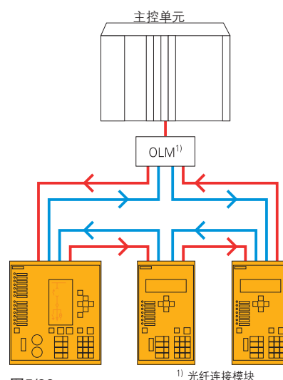
图5/88 PROFIBUS：光纤双环回路
