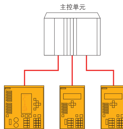
图5/87 IEC 60870-5-103：辐射形光纤连接
