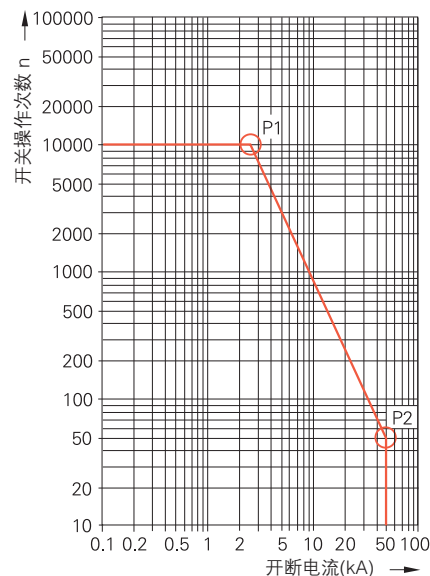
图 5/85: CB操作周期图表
