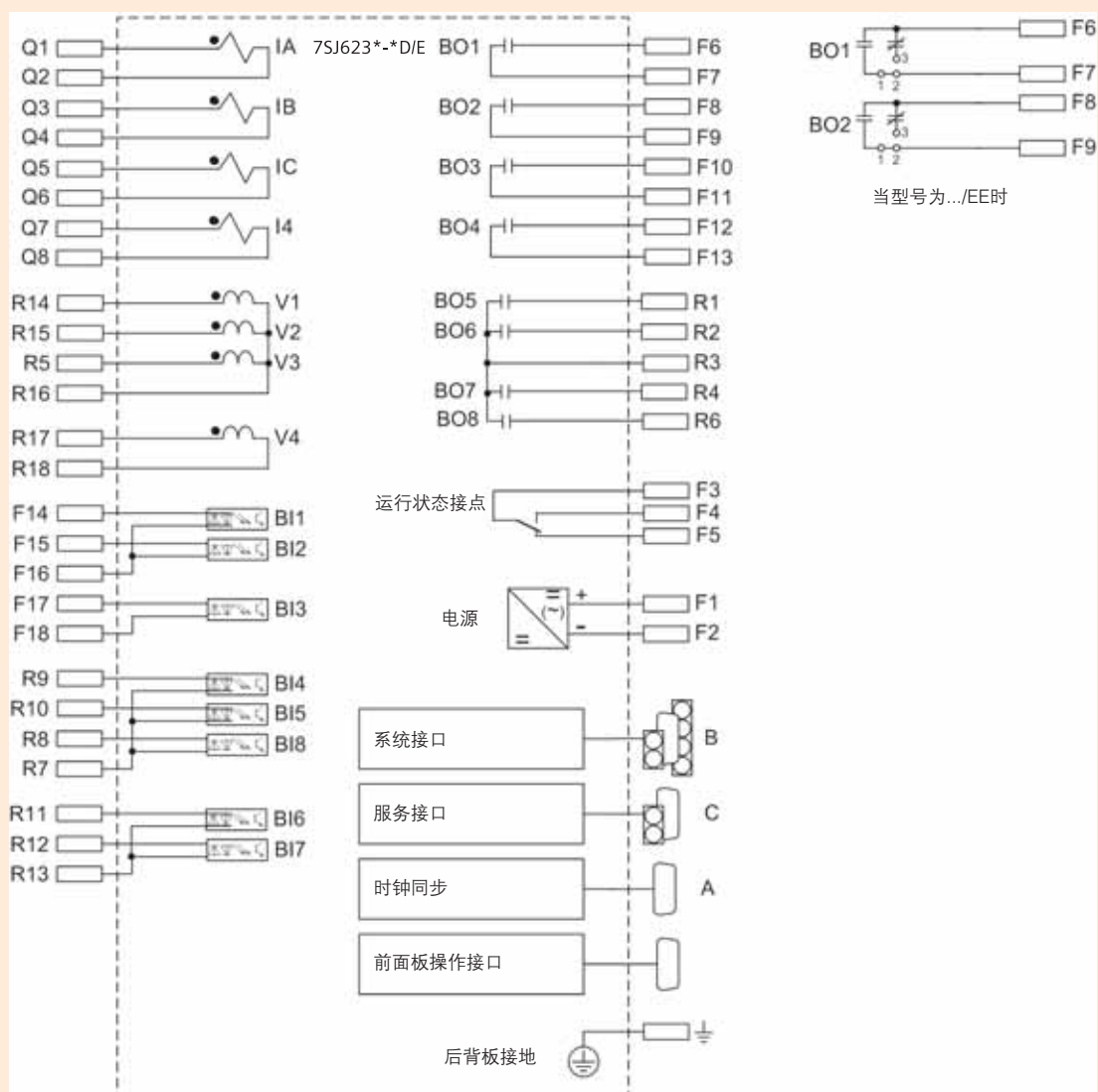
图5/104 7SJ623*-* DIE 接线图
