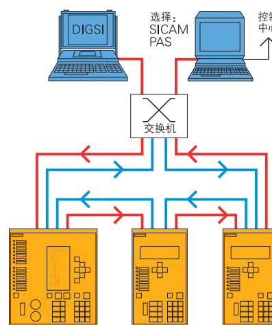
图5/89 由以太网、IEC 61850和光纤环网组成的站控总线
