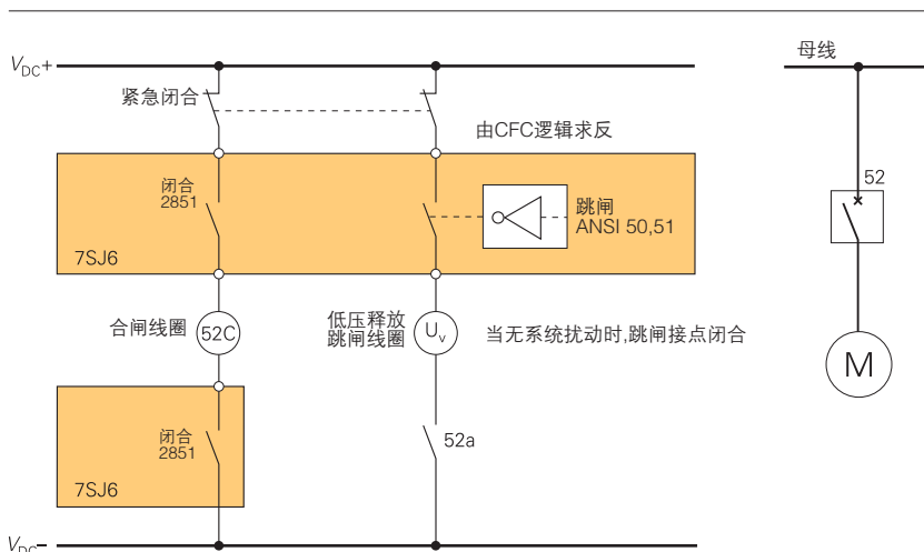
图5/99: 带闭锁接点的欠压释放 (跳闸信号50取反)
