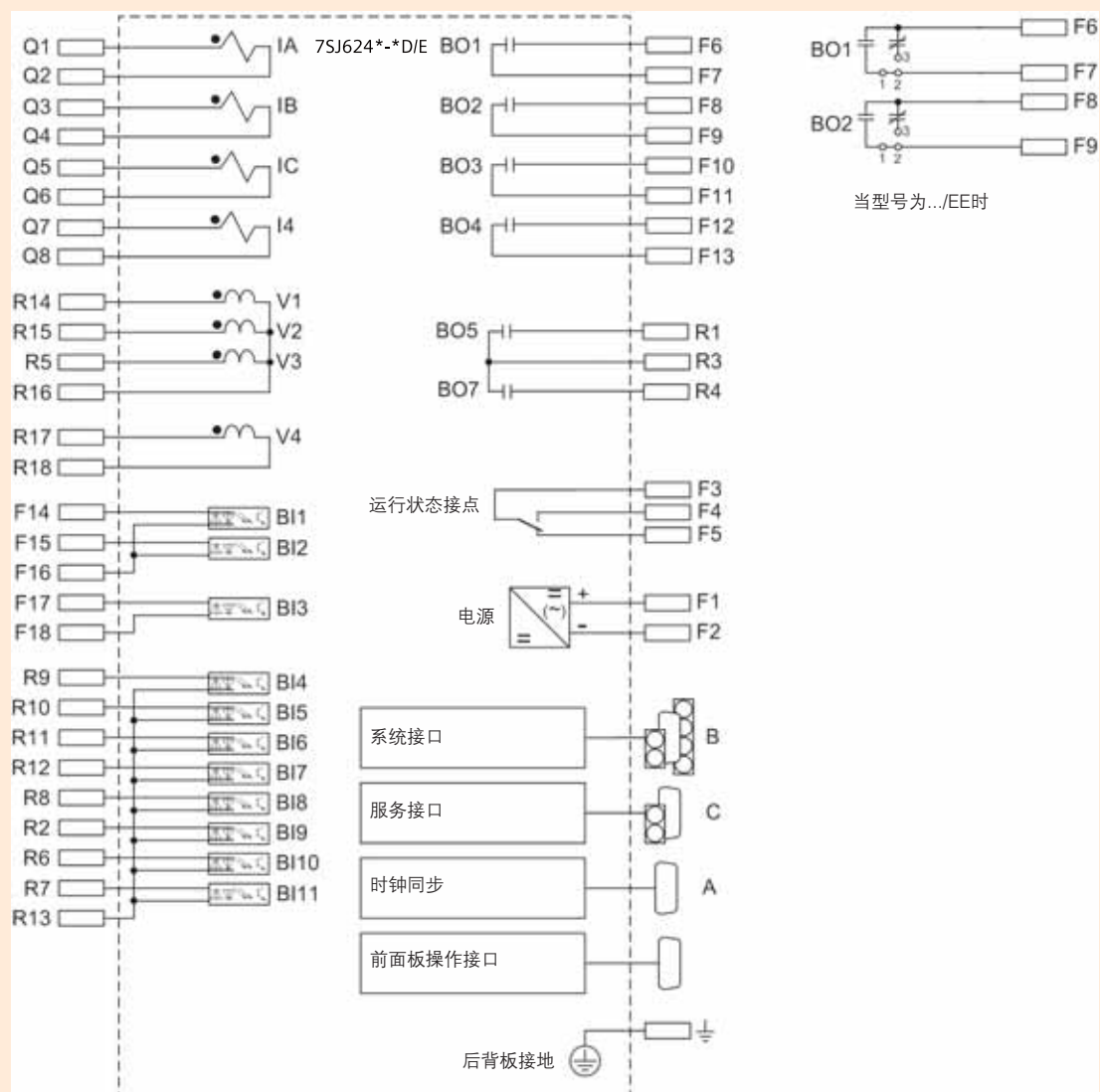
图5/104 7SJ624*-*/D/E 接线图
