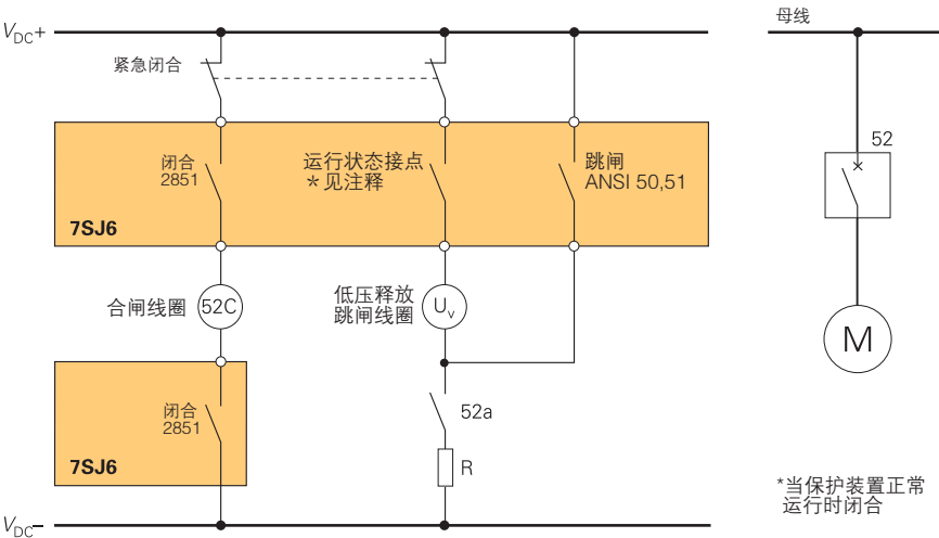
图5/98：带50，51接点的欠压释放
