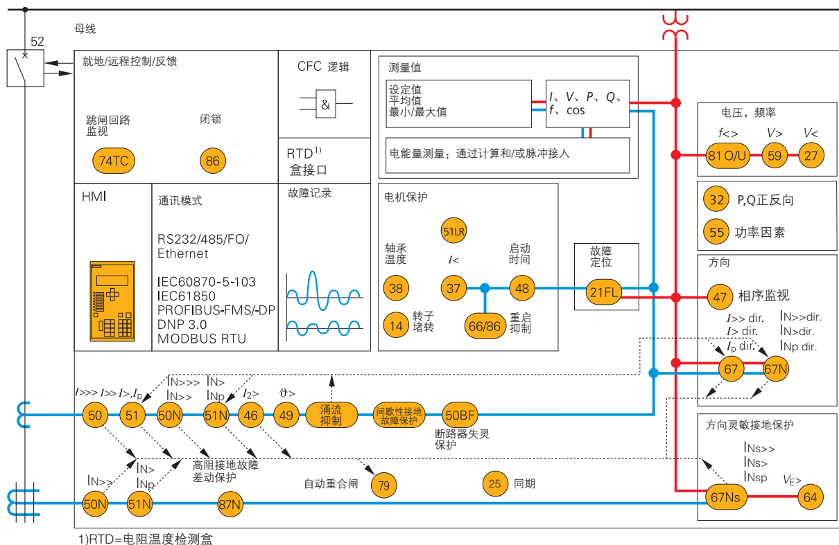
图5/77：功能图
