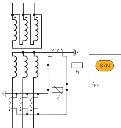
图5/83：高阻接地故障差动保护
