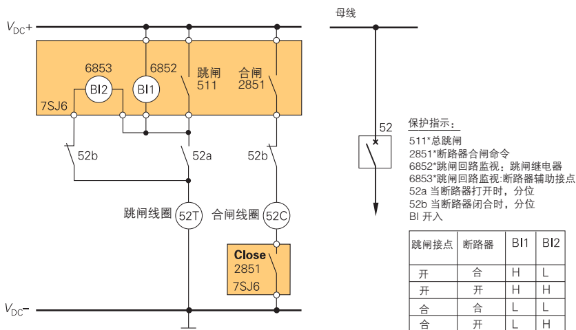
图5/100: 带两个开入量的跳闸回路监视
