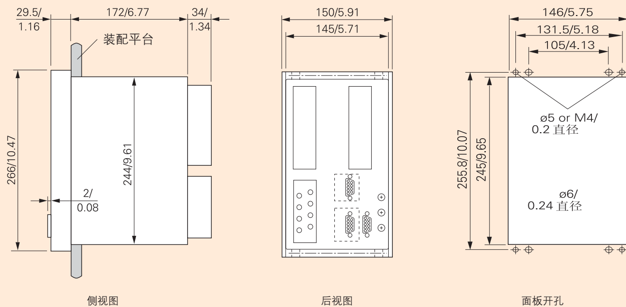
图16/22: 嵌入式安装/机柜式安装机架 (1/3 X19")
