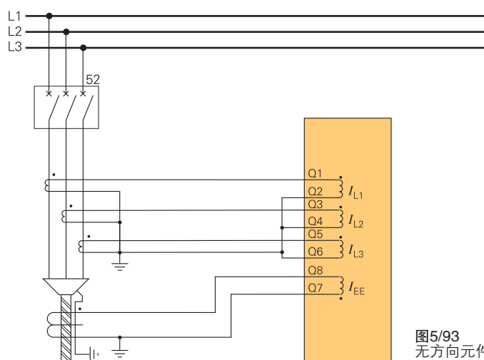
图5/92 无方向元件的残余电流回路
