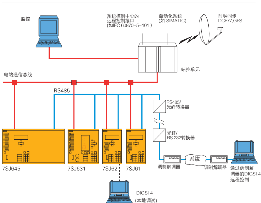
图5/90 系统解决方案/通讯
