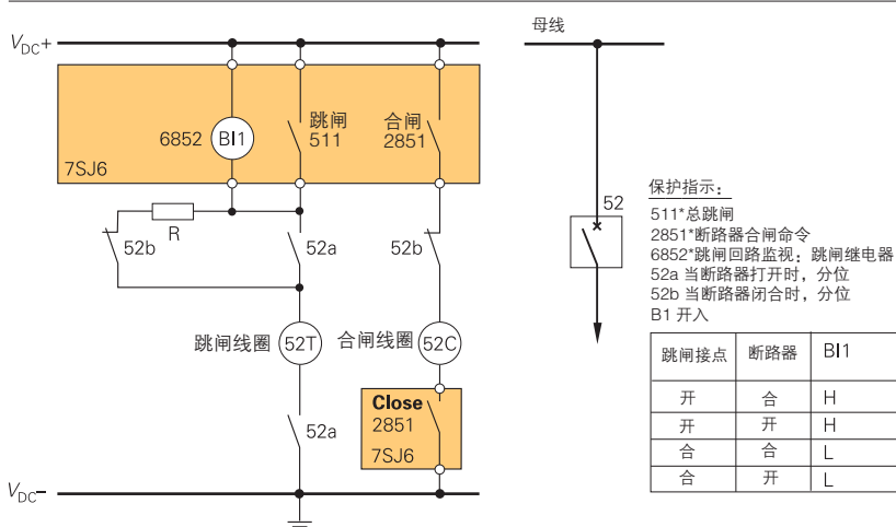
图5/101: 带一个开入量的跳闸回路监视
