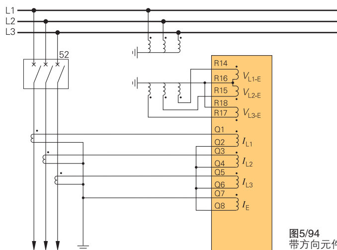
图5/93 无方向元件的灵敏接地电流检测
