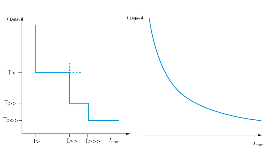
图 5/79: 定时限过流保护
