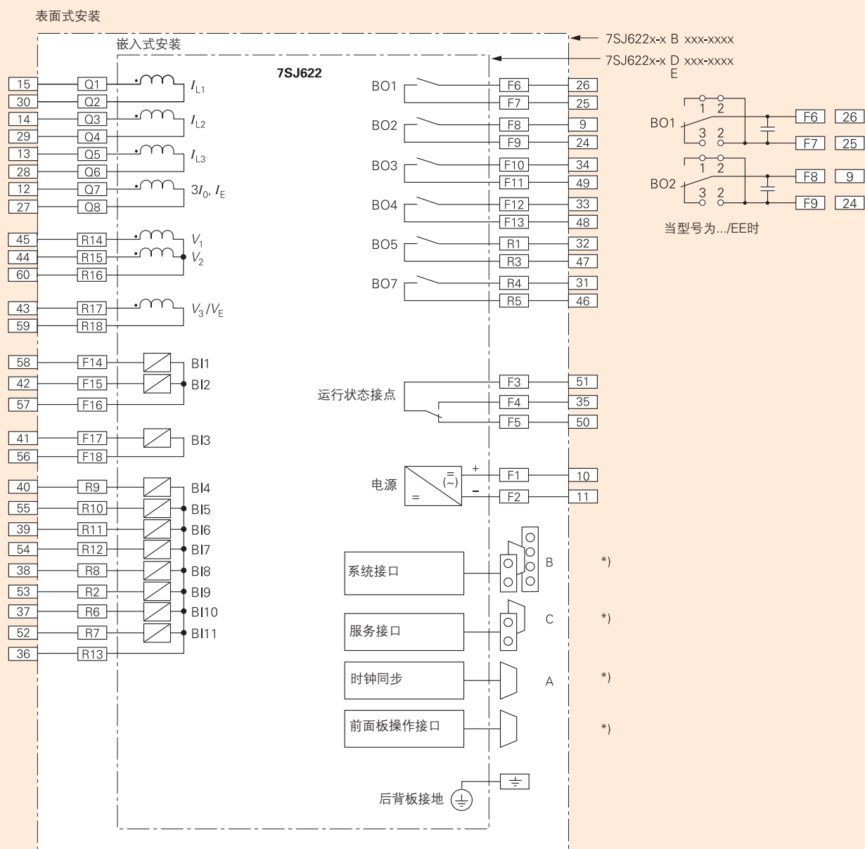
图5/103: 7SJ622接线图
