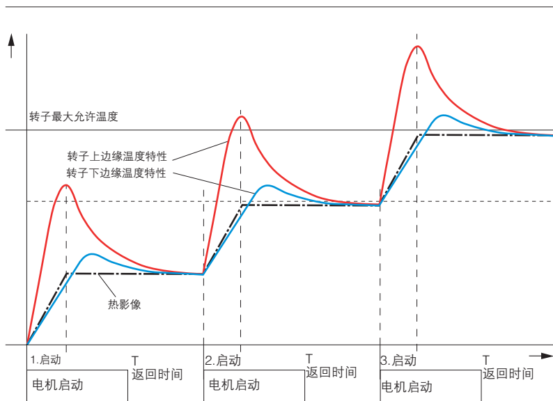
图 5/84：重启抑制特性
